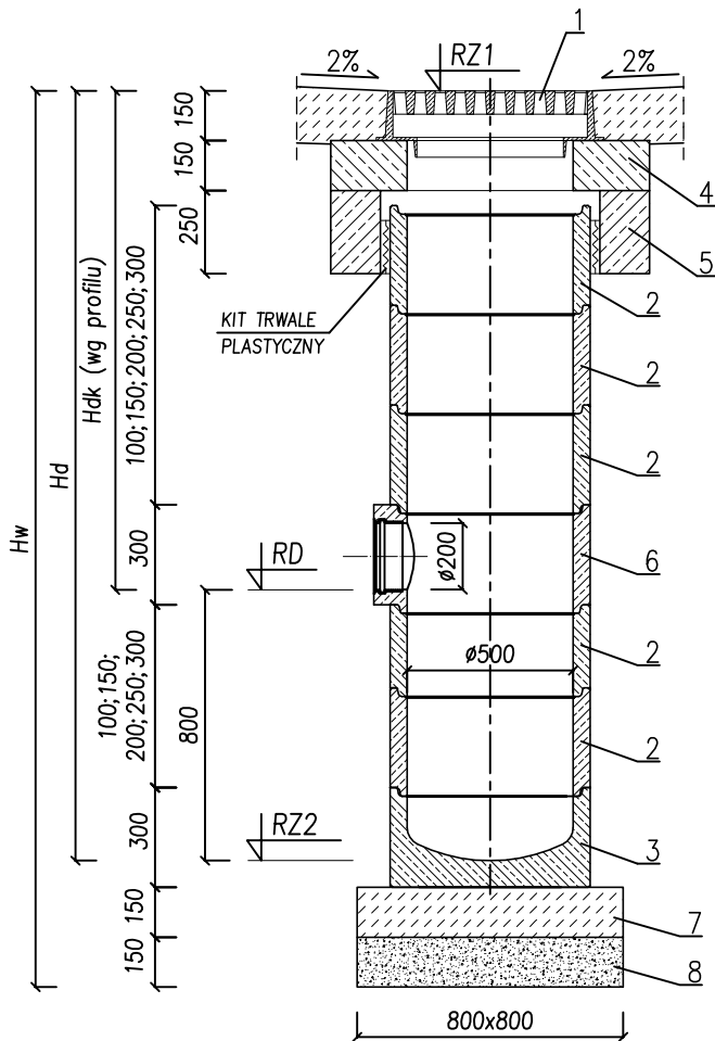
PRZĘKRÓJ A-A
