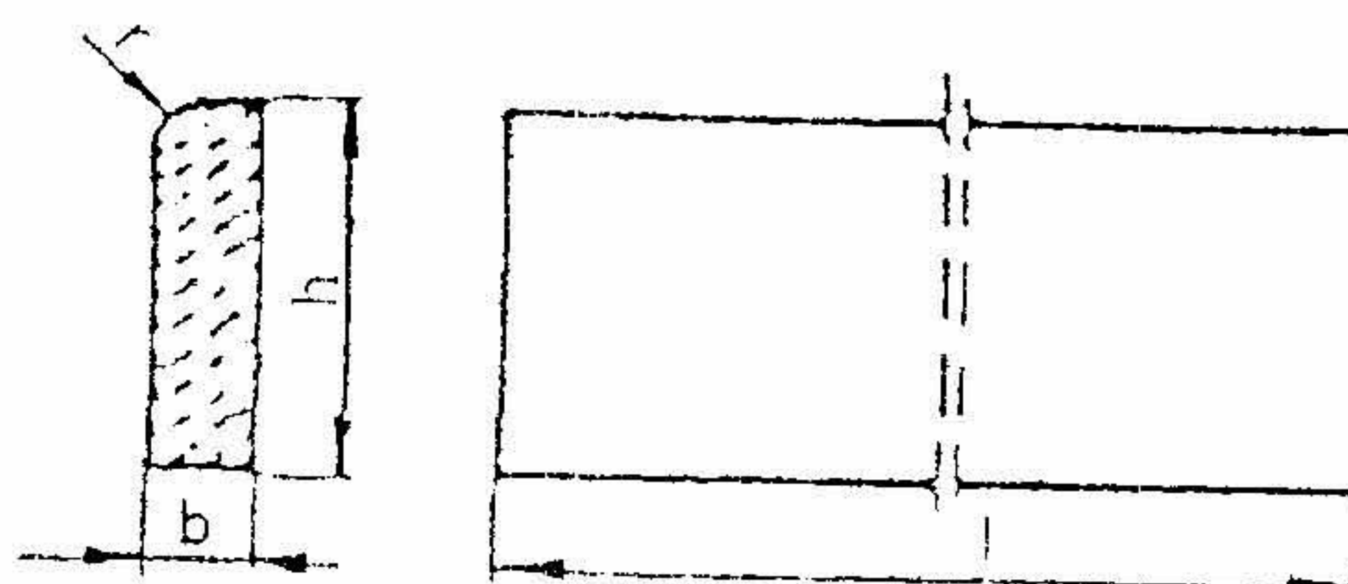
Rysunek 1. Kształt betonowego obrzeża chodnikowego
