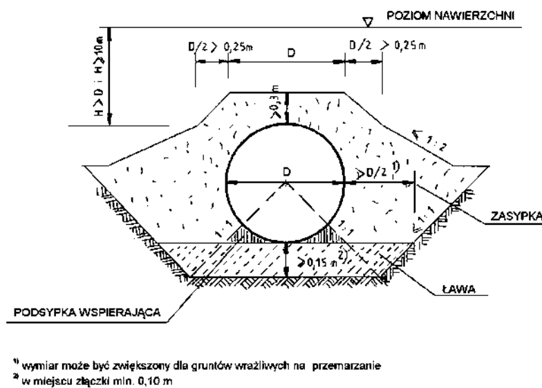
Rys. 8. Zasyпка nad przepustem jednorurowym
